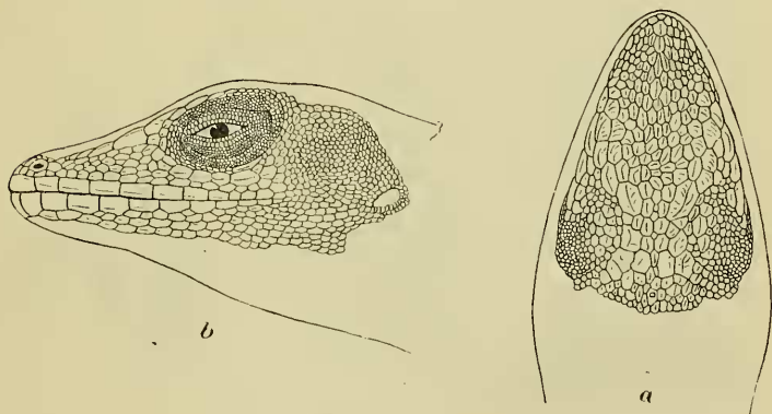
Anolis apollinaris .
